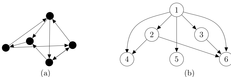
FIGURE 1 . (a) un graphe, (b) le graphe de la relation de divisibilité sur \{1, 2, 3, 4, 5, 6, \} : on a omis les boucles en chaque sommet, qui correspondent à la divisibilité de n par lui même.
