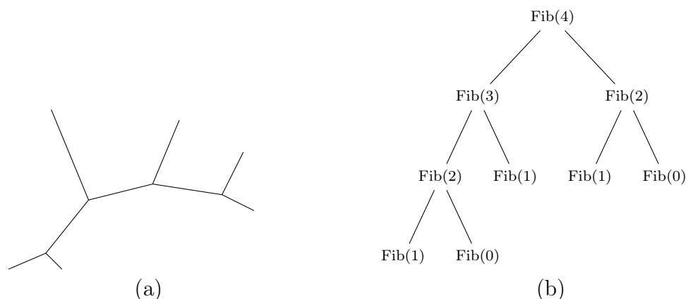
FIGURE 2 . (a) un arbre, (b) l'arbre des appels récursifs de la suite de Fibonacci.
