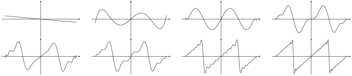
FIGURE 7 . Approximations de la fonction f_1 définie sur [-1, 1] par f_1(t) = t si |t| < 1/2 et f_1(t) = t - \text{sgn}(t) si |t| \geq 1/2 par la somme de polynômes de Chebyshev \sum_{n=0}^N t_n(f_1)T_n pour N = 2, 6, 10, 14, 18, 22, 50, 100 .
