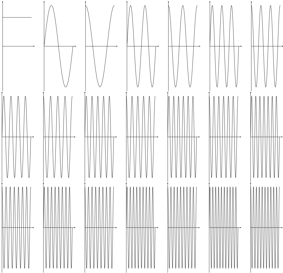
FIGURE 2 . Les fonctions cos/sinusoïdales E_n sur [0, 1] pour n = 0, \dots, 20 .
